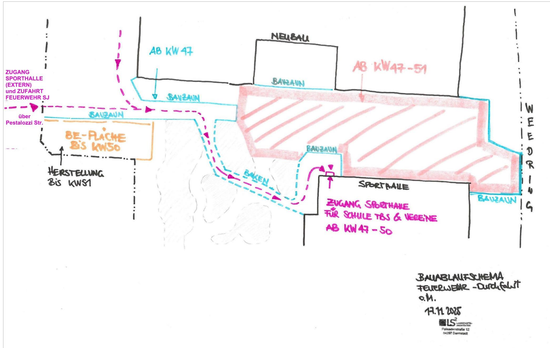
Lageplan-Skizze: Korridor / Wegeführung aus Richtung Pestalozzistraße
